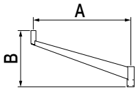
crosse TOP CLIP simple feu
