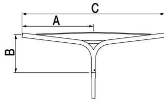
crosse PALAMA double feu
