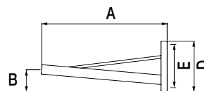
applique contre-feu / applique murale MUSA
