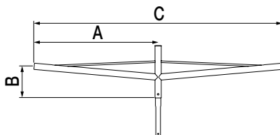
crosse MUSA double feu
